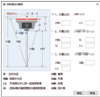
(获取基站仪器高)
