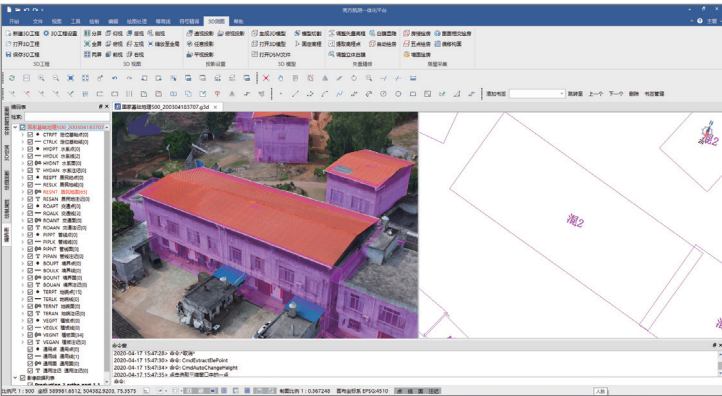
(三维测图功能图)
